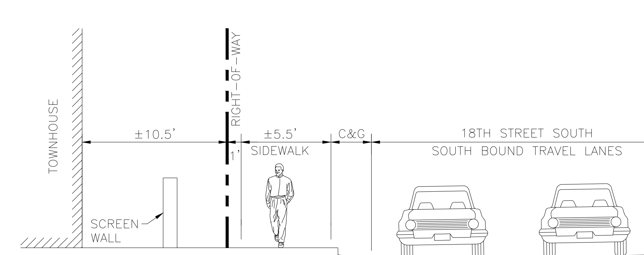
TYPICAL SECTION N.T.S.
